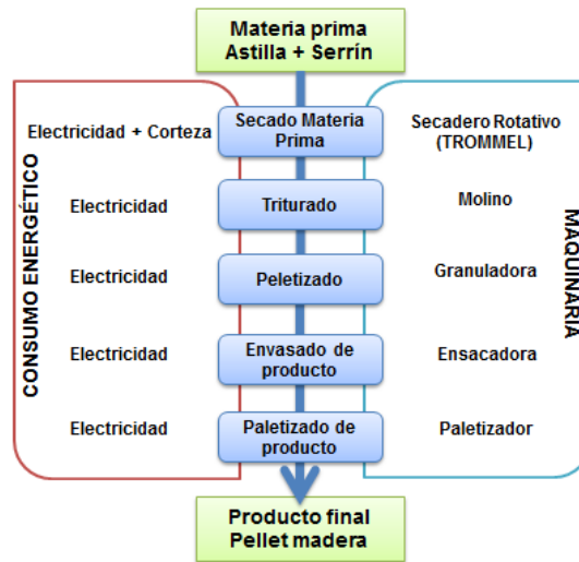
Figura 1. Diagrama de flujo de la fábrica de pellets
